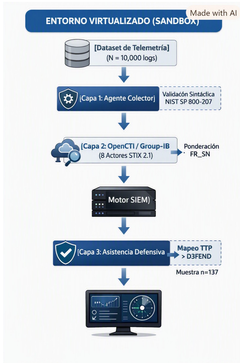
Figura 2: Arquitectura del Entorno Experimental Sandbox (Docker, SIEM y OpenCTI)
