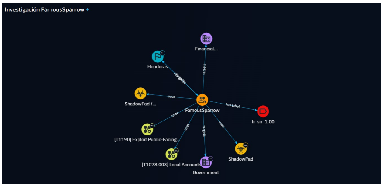
Figura 3: Grafo Relacional de Ciberinteligencia para el Actor FamousSparrow en OpenCTI (Estándar STIX 2.1)
